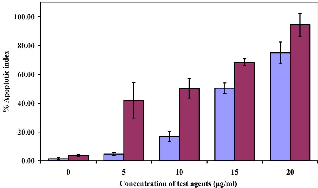
■ xanthorrhizol ■ xanthorrhizol-curcumin
